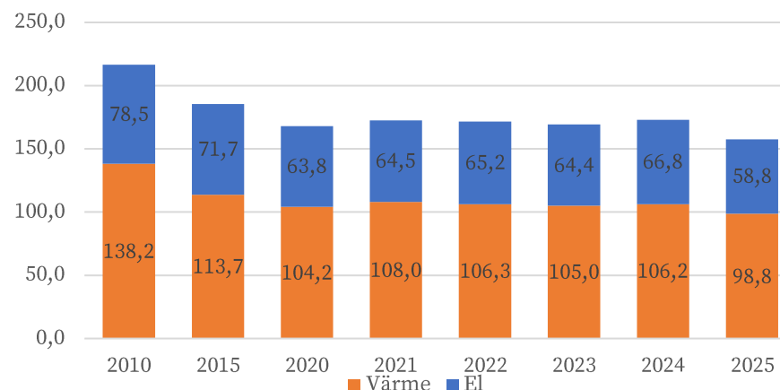
Figur 12. Energianvändningen i Skövde kommuns fastigheter från 2010 till 2025 (kWh/m²).
