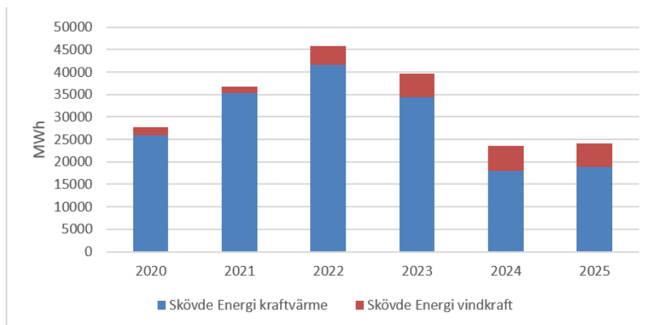
Figur 11. Produktion av el av Skövde Energi
