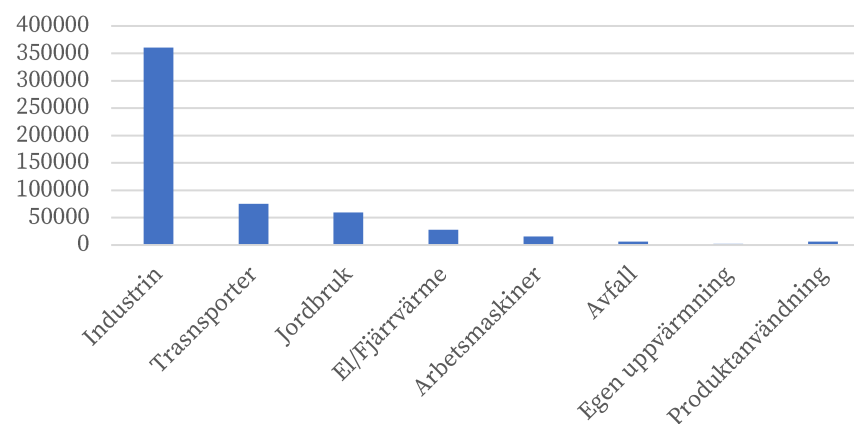
Figur 6, Skövdes växthusgasutsläpp 2024. Nationella Emissionsdatabasen
