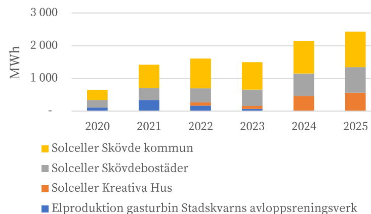
Figur 10. Produktion av solenergi inom kommunkoncernen, utöver produktion hos Skövde energi. Skövde kommun
