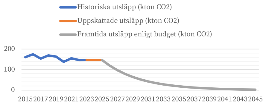
Figur 5, Västra Götalands läns koldioxidbudget, Skövde kommuns energi- och klimatplan
