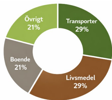
Figur 7, Hushållens konsumtionsbaserade utsläpp i Sverige. Naturvårdsverket
